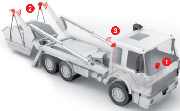
1 Wiegeelektronik
