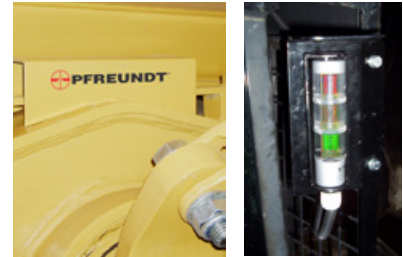
2 Eléments de mesure DW-3 avec voyant de charge LED
