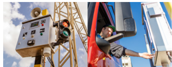
Outdoor-Terminal mit Ampelanlage
