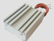
Chauffage du coffret de distribution
